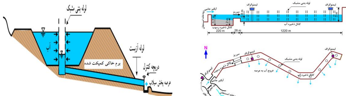
شکل (۲): یلان کانال‌های ذخیره و خروجی سیفون معکوس
