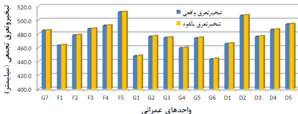
شکل (۲): مقایسه بین متوسط تبخیر تعرق واقعی و پتانسیل تجمعی در واحدهای عمرانی حوضه دشت سفیدرود
