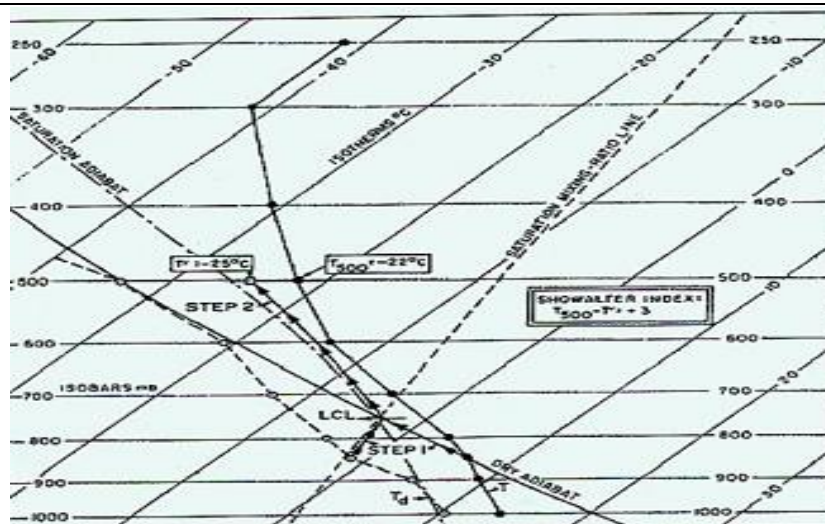
شکل (۱): تعیین مرحله به مرحله شاخص شولتر بر نمودار اسکیت
