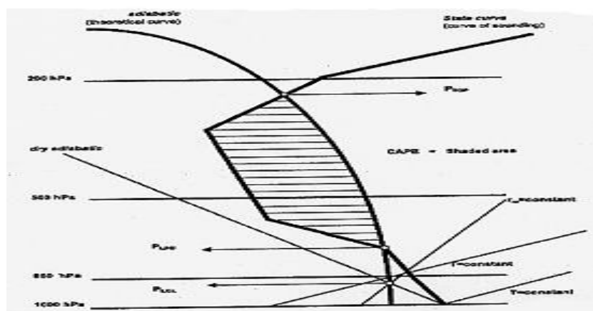
شکل (۲): محاسبه مقدار انرژی پتانسیل در دسترس همرفتی به کمک نمودار اسکیوتی
