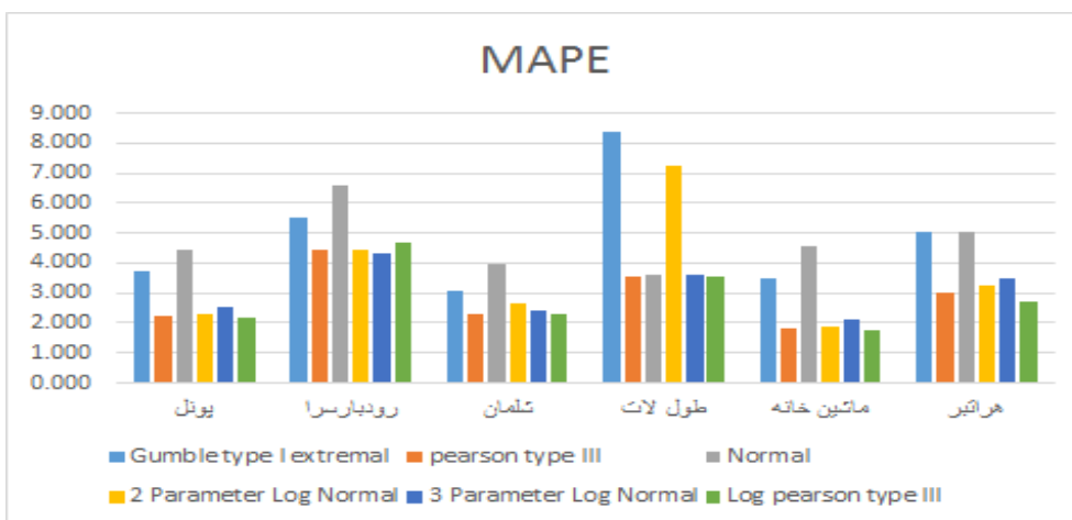
شکل (۳): مقایسه توزیع‌های مورد استفاده با شاخص MAPE طی دوره آماری ۵۰ ساله
