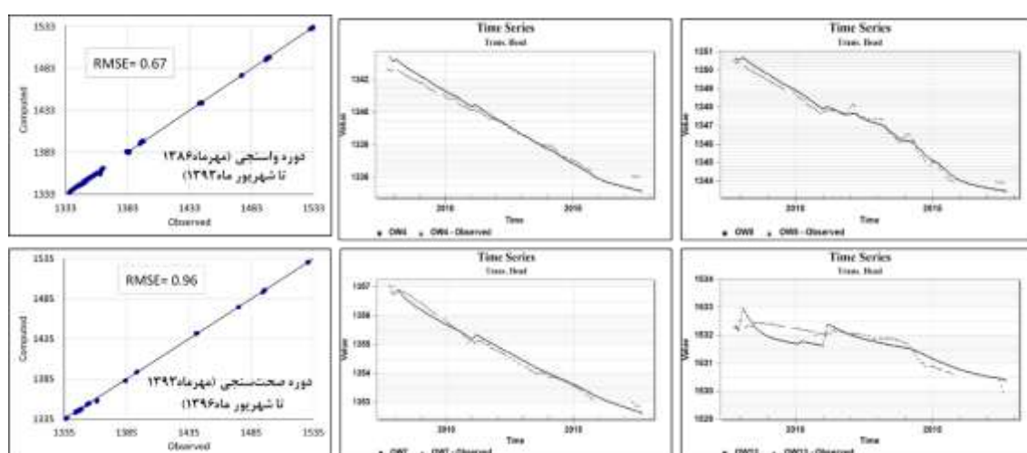
شکل (۵): مقایسه مقادیر تراز سطح آب مشاهده‌ای و محاسباتی در طی دوره واسنجی و صحت سنجی مدل جریان آب زیرزمینی خاش
