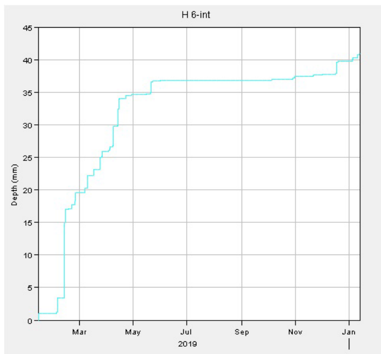
شکل (۶): نمودار میانگین تلفات تجمعی سالیانه زیر حوزه H 6-int
