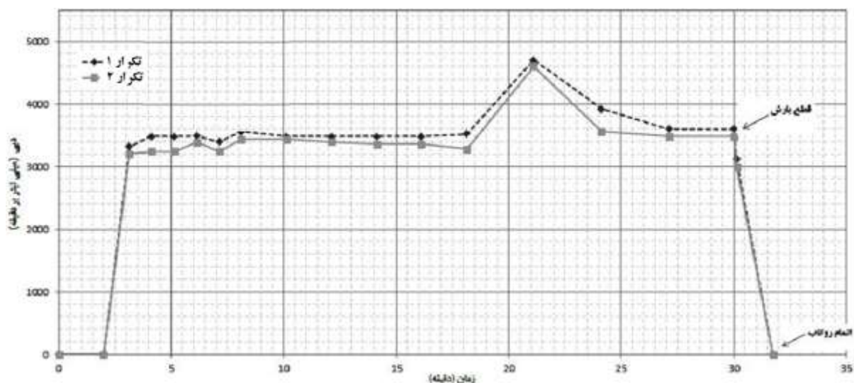
شکل (۵): نمودار تغییرات دبی در مدت ۳۰ دقیقه در شیب ۱۲ درصد خاک سراب ننیز
