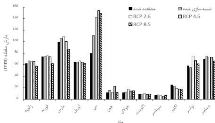
شکل (۲): میانگین بارش ماهانه ۱۹۹۲-۲۰۱۹ و ۲۰۲۱-۲۰۵۰ تحت تأثیر سناریوهای RCP2.6، RCP4.5 و RCP8.5
