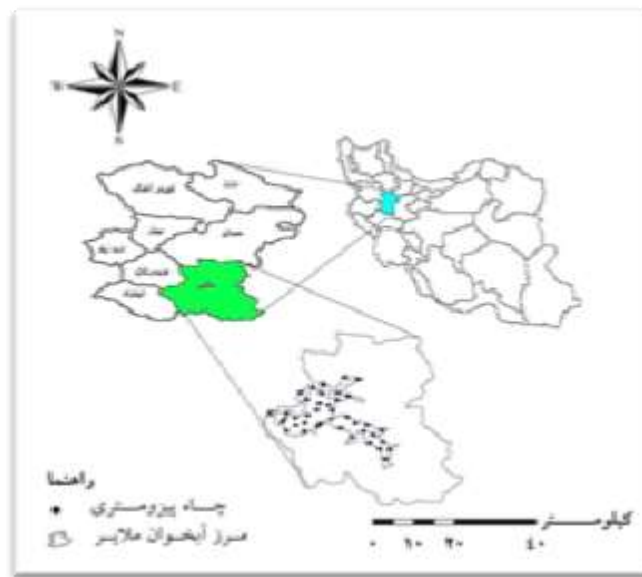
شکل (۱): موقعیت دشت ملایر و چاه‌های پیرومتری
