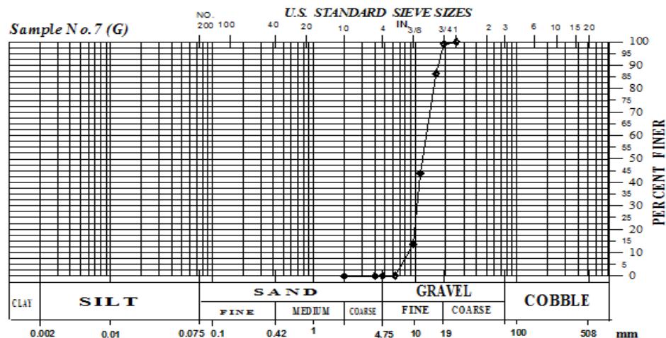
شکل (۵): منحنی دانه‌بندی شن مورد استفاده به‌عنوان پوشش محافظ در کرت‌های آزمایشی
