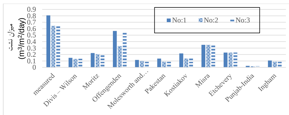
شکل (۸): مقایسه نشت برآورد شده از روش‌های مختلف تجربی با نشت اندازه‌گیری شده در کانال حسن‌آباد
