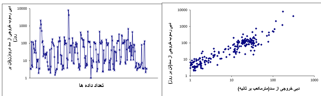
د- تغییرات دبی رسوب خروجی از سد
