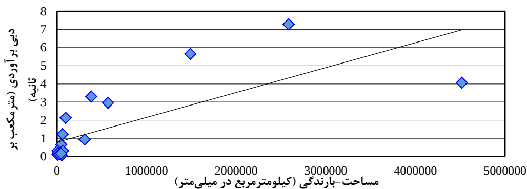
شکل (۶): رابطه میان دبی متوسط جریان و مساحت حوضه-بارندگی (رابطه ۱۴)
