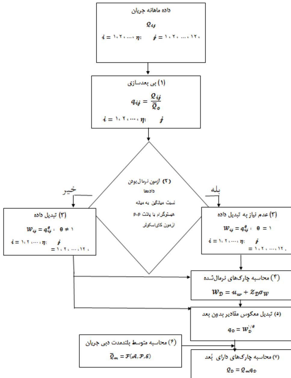
شکل (۲): مراحل مدل‌سازی غیرخطی منحنی تداوم جریان (اقتباس از Burgan &amp; Aksoy, 2020)
