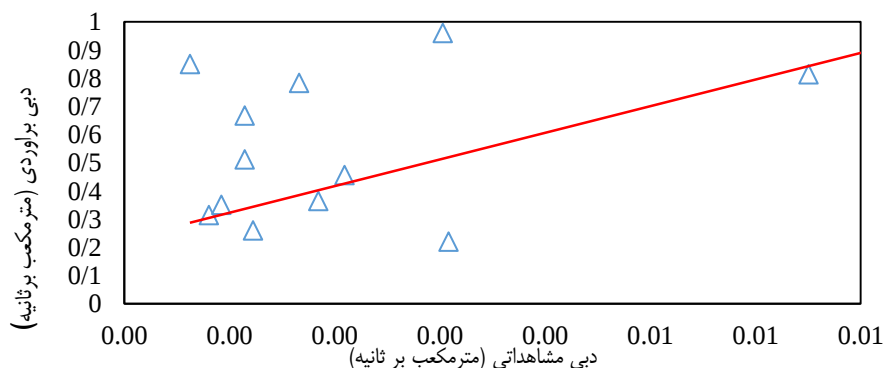
شکل (۷): رابطه مقدار مشاهده شده و برآورد شده دبی متوسط برای ایستگاه آلاذیزگه
