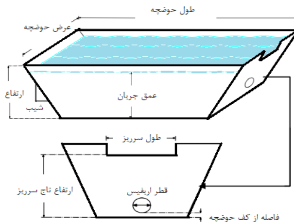
شکل ۴- طرح شماتیک حوضچه تاخیری ذوزنقه‌ای با خروجی اریفیس دایره‌ای و سرریز مستطیلی
