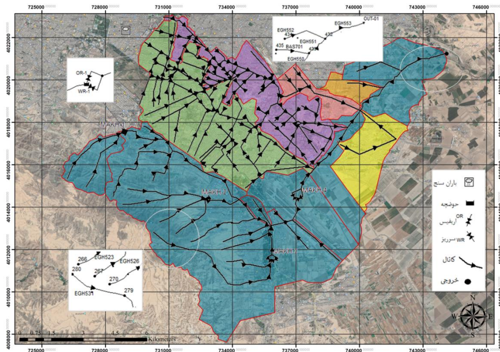
شکل ۳- مدل‌سازی شبکه و حوضچه‌های تاخیری در محیط SWMM 5.0
