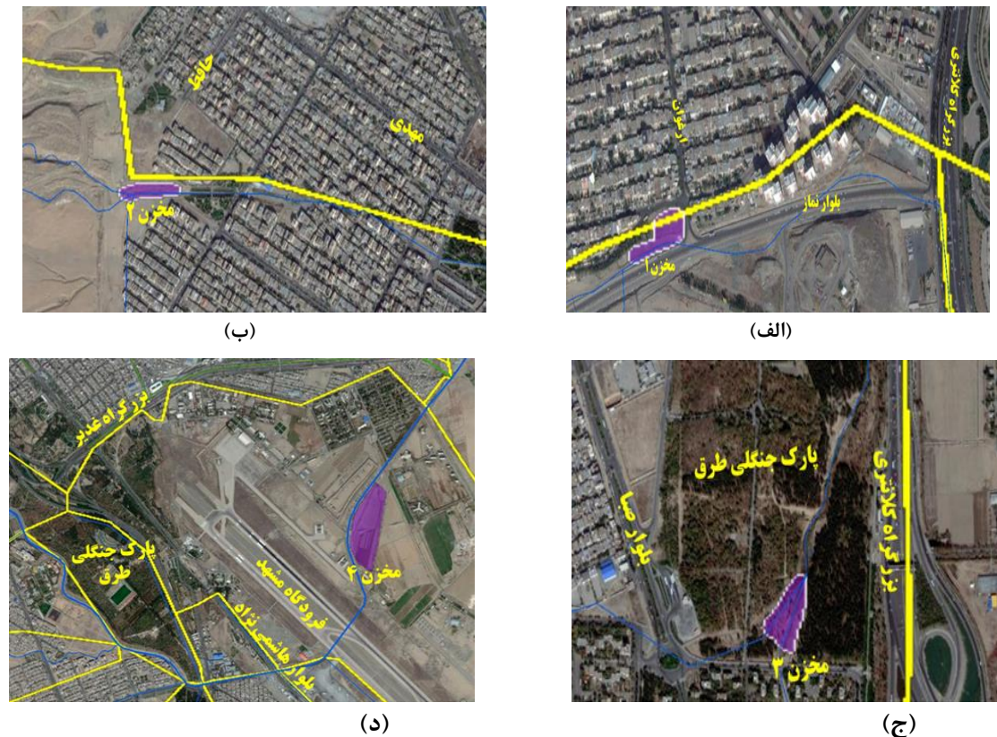
شکل ۸- الف) جانمایی مخزن ۱ در بلوار نماز، سرشاخه ذکریا، ب) جانمایی مخزن ۲ سرشاخه قائم، ج) جانمایی مخزن ۳ داخل پارک طرق، سرشاخه ابوذر و د) جانمایی مخزن ۴ در فرودگاه مشهد، مسیر اقبال شرقی Figure 8- a) Placement of delay pond 1 in Namaz Boulevard, Zakaria branch, b) Placement of the delay pond 2 Zakaria branch, and c) Placement of delay pond 3 inside Torogh Park, Abu Dhar branch and d) Placement of delay pond 4 at Mashhad Airport, East Eghbal Flood Way
