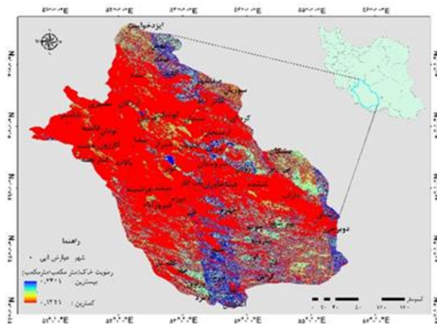
شکل (۴): پراکندگی رطوبت خاک در سال پربارش
