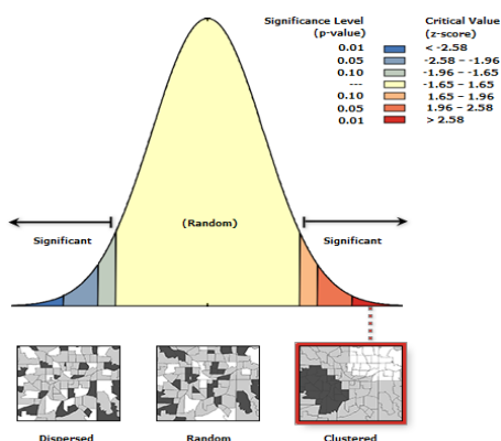
شکل (۶): نحوه خوشه‌بندی ناهنجاری رطوبت
