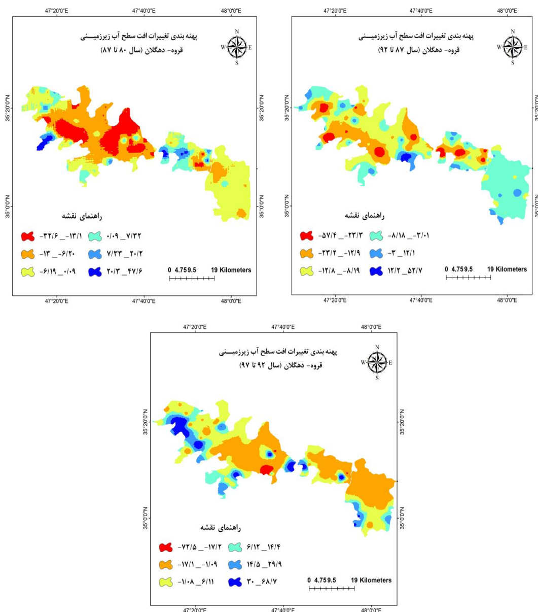
شکل ۴- پهنه‌بندی تغییرات افت آب زیرزمینی (بر حسب سانتی‌متر) در سه دوره زمانی Figure 4- Zoning of changes in groundwater drop (cm) in three time periods
