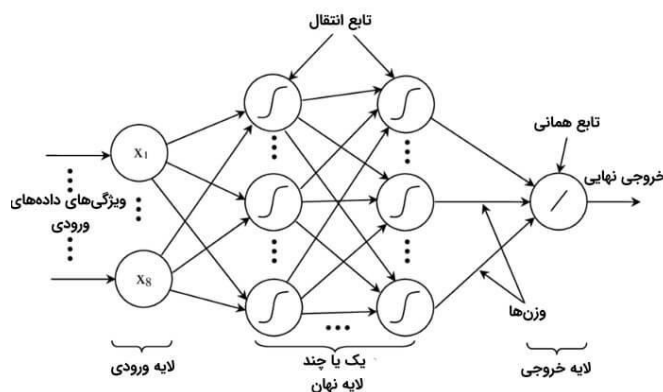
شکل ۳- ساختار یک شبکه عصبی مصنوعی پرسپترون چند لایه
