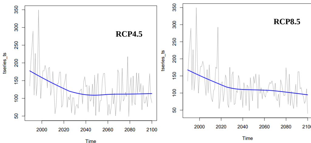
شکل ۱۰- منحنی سری زمانی بارش (میلی‌متر) شبیه‌سازی شده زیرحوزه آبخیز اولنگ برای دوره ۱۹۸۹-۲۱۰۰ تحت سناریوهای RCP4.5 و RCP8.5
