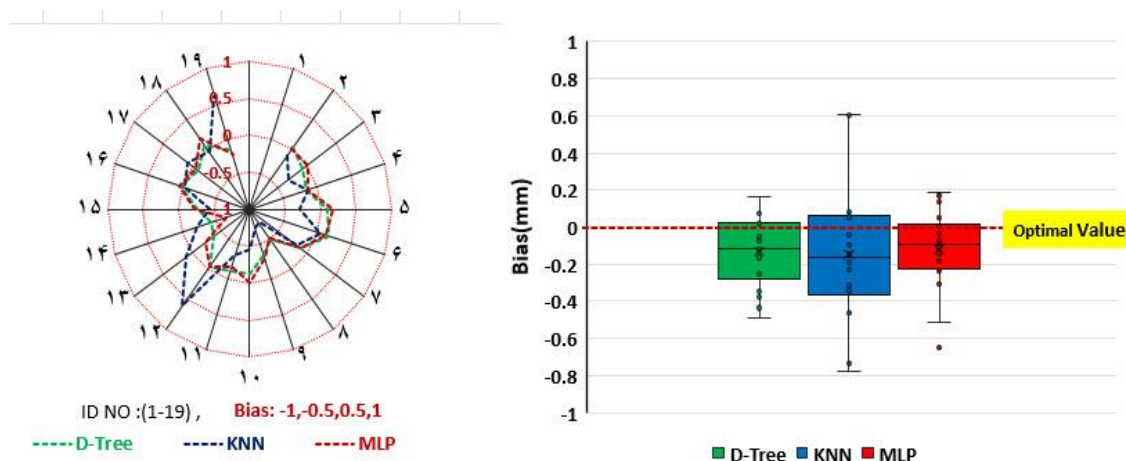
شکل ۴- مقایسه شاخص آماری سوگیری بارش تخمینی داده‌های آزمایشی و مقادیر ایستگاهی با استفاده از الگوریتم‌های مورد استفاده Figure 4- Comparison of the statistical bias index of the estimated precipitation of experimental data and station values using the used algorithms
