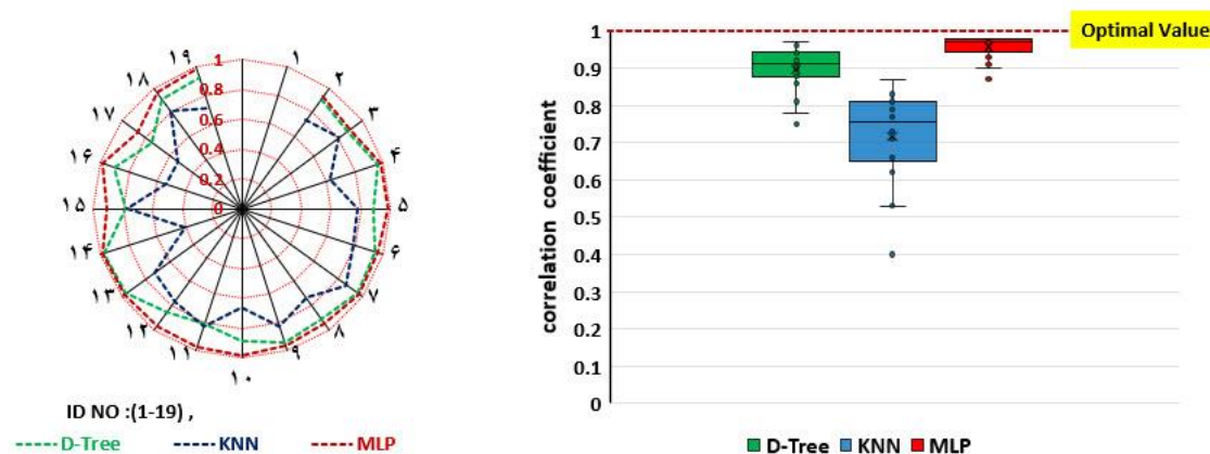
شکل ۲- مقایسه شاخص آماری ضریب همبستگی بارش تخمینی داده‌های آزمایشی و مقادیر ایستگاهی با استفاده از الگوریتم‌های مورد استفاده
