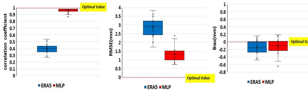
شکل ۵- مقایسه شاخص‌های آماری بارش روزانه ERA5 واسنجی شده برای ایستگاه‌های شاهد
