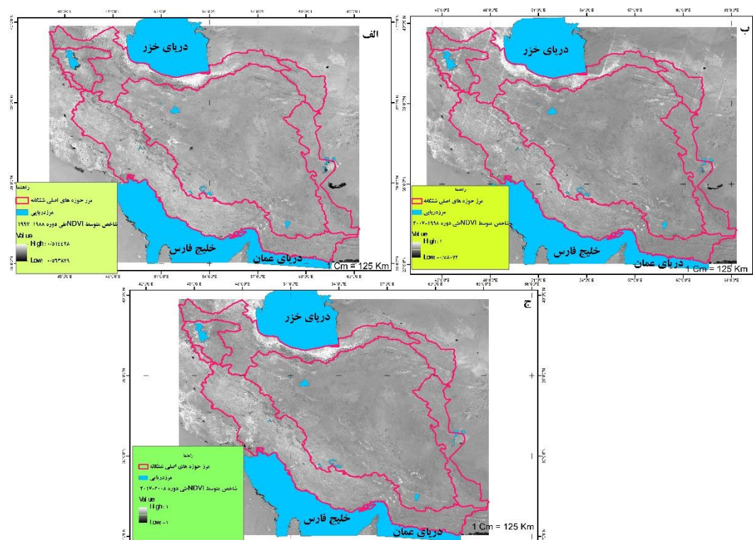
شکل ۳- شاخص تفاوت پوشش گیاهی نرمال شده (NDVI) در زیرحوضه‌های آبگیر اصلی در سه دوره زمانی ۱۰ ساله
