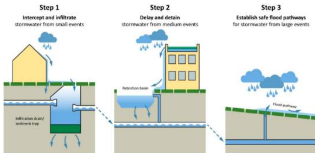
شکل ۲- راهبرد سه مرحله ای نروژ برای مدیریت آب سیلابی (Thodesen et al., 2022) Figure 2- Norway's three-stage strategy for flood water management
