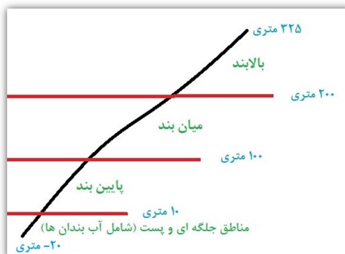
شکل ۴- طبقات ارتفاعی در منطقه مورد مطالعه Figure 4- Altitude ranges in the studied area
