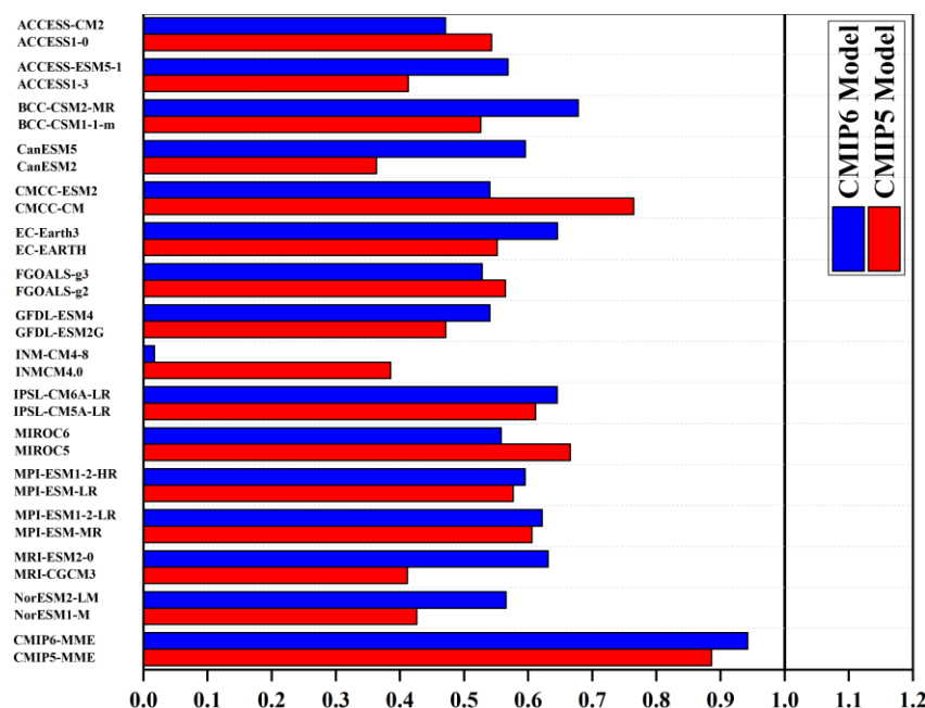
شکل ۳. معیار TSS بارش ماهانه شبیه‌سازی شده طی دوره ۲۰۰۵-۱۹۷۶ در ایران تحت مدل‌های CMIP6 (آبی) و CMIP5 (قرمز) Figure 3. Taylor skill scores of simulated monthly precipitation during the period 1976-2005 in Iran under CMIP6 (blue) and CMIP5 (red) models
