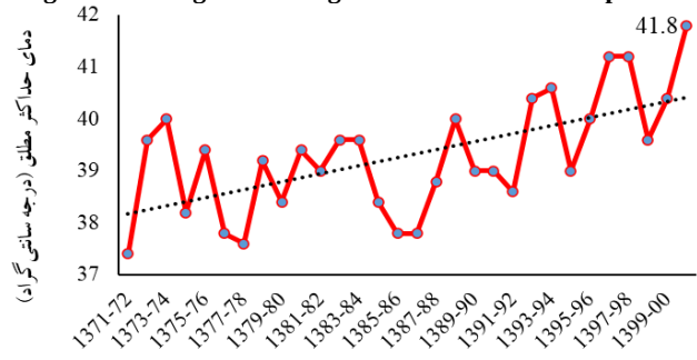
شکل ۹- تغییرات دمای حداکثر مطلق طی سنوات مختلف
