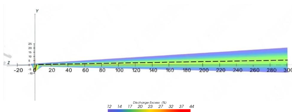
شکل ۴- نمای افقی تغییرات غلظت در مسیر هاله آلودگی
