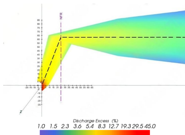
شکل ۸- نمای افقی تغییرات غلظت پساب شور در مسیر هاله آلودگی قبل اسلک
