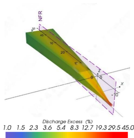
شکل ۷- نمای افقی تغییرات غلظت شوری در مسیر هاله آلودگی در اسلک
