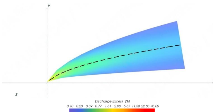
شکل ۲- نمای افقی تغییرات غلظت شوری در مسیر هاله آلودگی
