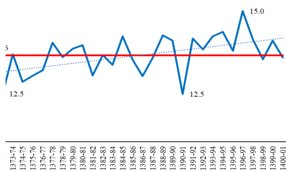
شکل ۸- تغییرات متوسط دمای سالانه Figure 8- Average annual temperature changes
