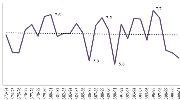
شکل ۷- تغییرات دمای میانگین حداقل سالانه Figure 7- Changes in average annual minimum temperature
