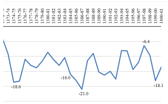
شکل ۱۰- تغییرات دمای حداقل مطلق طی سنوات مختلف Figure 10- Changes in absolute minimum temperature over different years
