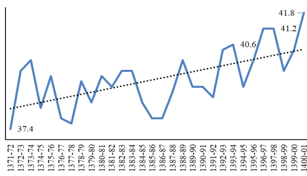
شکل ۹- تغییرات دمای حداکثر مطلق طی سنوات مختلف Figure 9- Changes in absolute maximum temperature over different years
