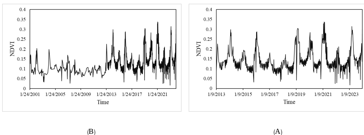
شکل ۳- تغییرات مقادیر NDVI در منطقه جنگل‌کاری شده (الف: بعد از جنگل‌کاری و ب: دوره مورد مطالعه) Figure 3- Changes in NDVI values in the afforested area (A: Post-afforestation, B: Study period)
