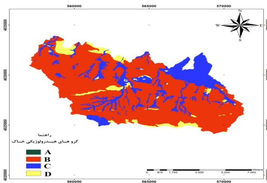
شکل (۴): نقشه گروه‌های هیدرولوژیک حوزه رود سراب خوشاب
