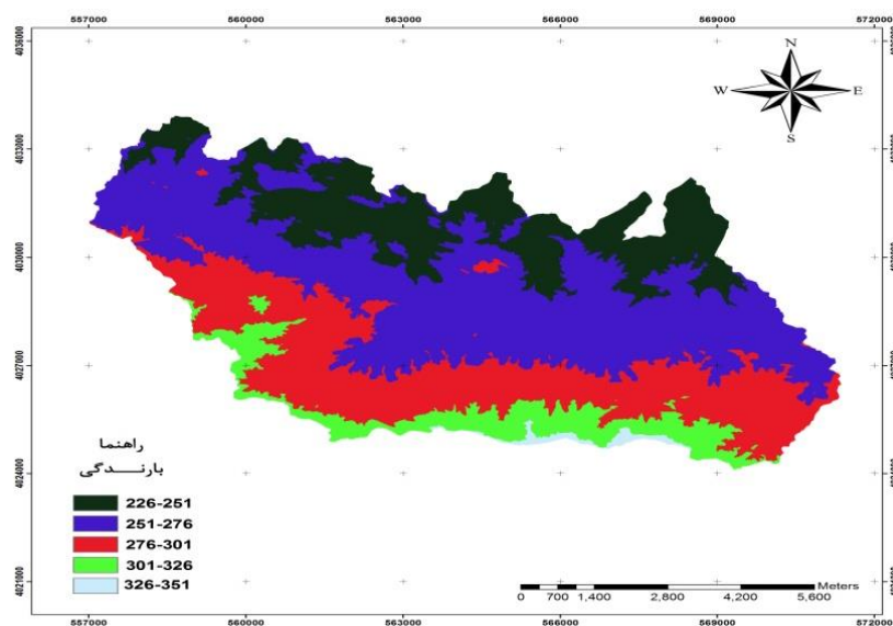
شکل (۷): نقشه بارندگی حوزه آبخیز رودسرآب خوشاب
