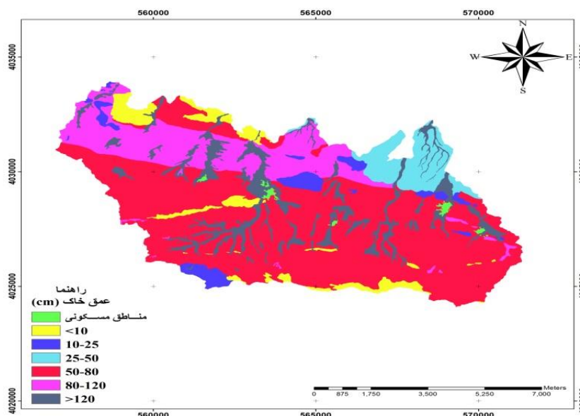
شکل (۶): نقشه عمق خاک حوزه آبخیز رود سراب خوشاب
