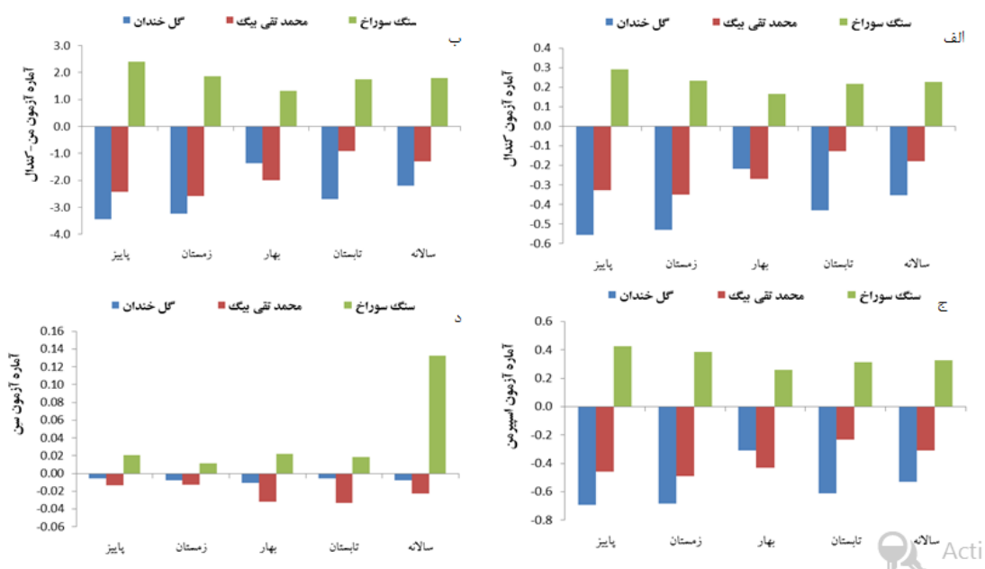
شکل (۳): نتایج آزمون‌های روند برای سری‌های سالانه و فصلی جریان رودخانه در ایستگاه‌های مورد مطالعه، الف) کندال ب) من-کندال ج) اسپیرمن د) سن
