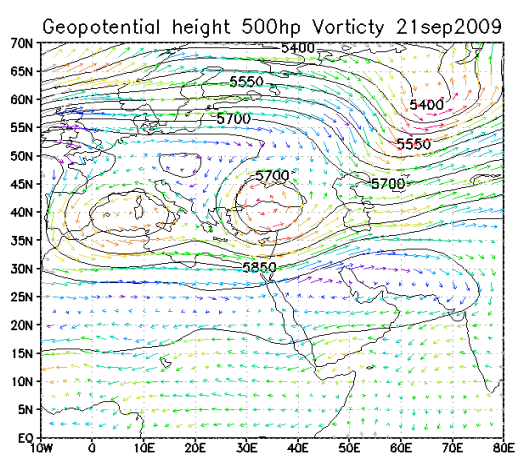
شکل (۶): الگوی سینوپتیکی هوای تراز سطح ۵۰۰ میلی‌بار ۲۱ سپتامبر
