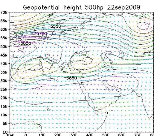
شکل (۸): الگوی سینوپتیکی هوای تراز سطح ۵۰۰ میلی‌بار ۲۲ سپتامبر
