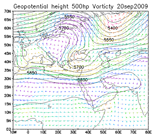
شکل (۴): الگوی سینوپتیکی هوای تراز سطح ۵۰۰ میلی‌بار ۲۰ سپتامبر
