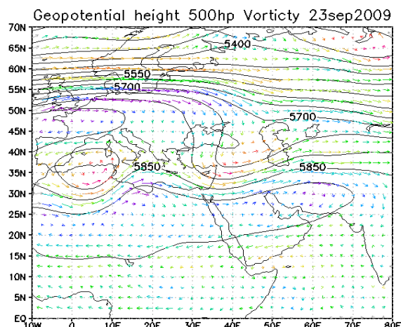
شکل (۱۰): الگوی سینوپتیکی هوای تراز سطح ۵۰۰ میلی‌بار ۲۳ سپتامبر شکل (۱۱): الگوی سینوپتیکی هوای تراز سطح ۱۰۰۰ میلی‌بار ۲۳ سپتامبر
