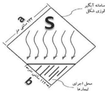
شکل (۳): ابعاد سطوح سامانه آبیگر لوزی شکل
