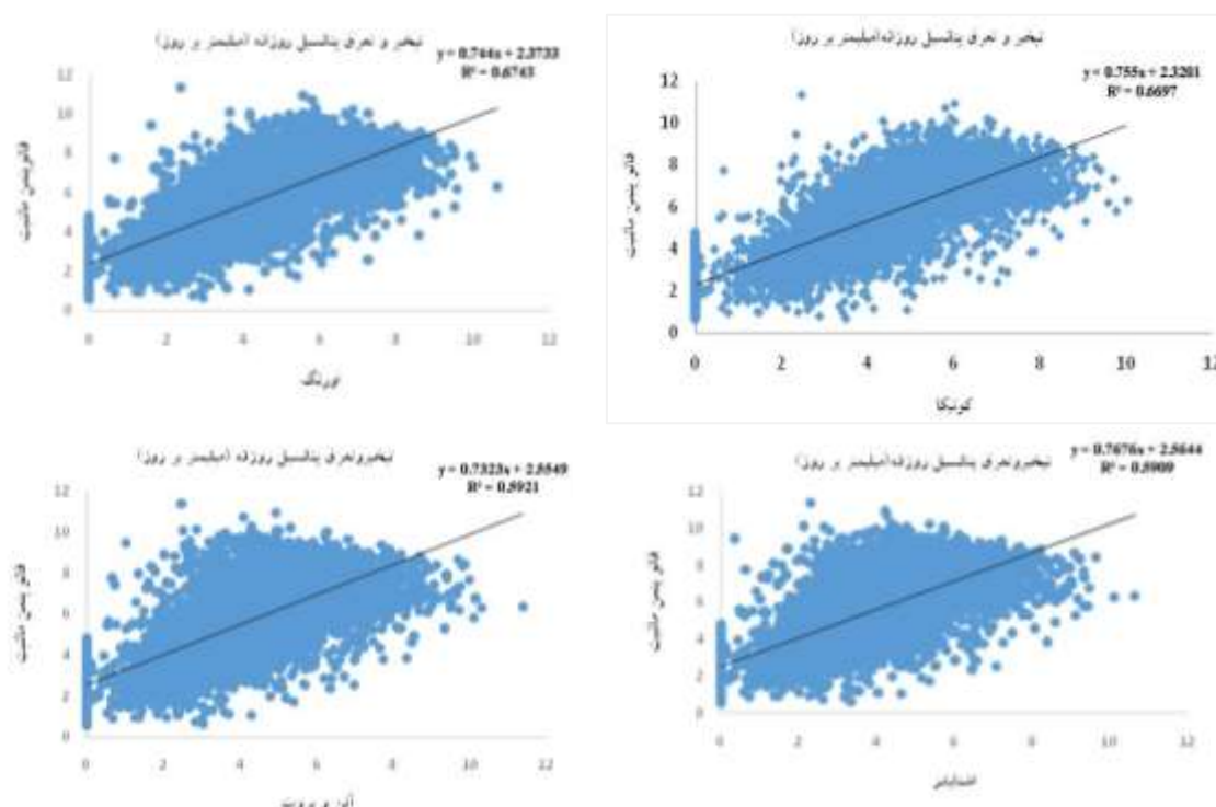
شکل (۳): مقایسه مقادیر روزانه ETo، محاسبه شده از مدل‌های برپایه ضریب تشت و روش استاندارد FPM (۱۳۹۵-۱۳۷۷)
