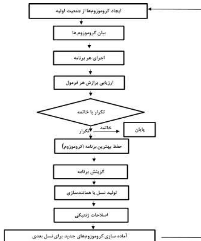
شکل (۲): فلوچارت الگوریتم بیان ژن
