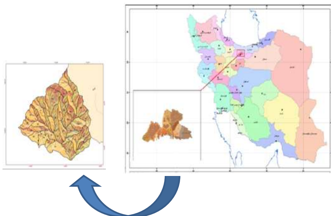
شکل (۱): نمایی از موقعیت حوضه دامنه جنوبی البرز (وردیج) محدوده مورد پژوهش
