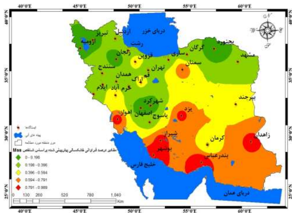
شکل (۷): بهینه‌بندی خشکسالی در سال‌های شبیه‌سازی شده بر اساس مدل M.S.S. در دوره آماری (۲۰۱۹-۲۰۲۳)
