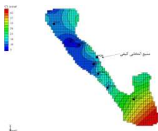
شکل (۴): نقشه غلظت اولیه کلر در مدل MT3DMS در مدل آب زیرزمینی خاش (یکای میلی گرم در لیتر)
