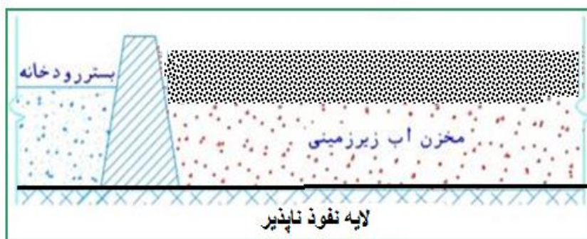
شکل (۲): تصویر شماتیک نمای کلی سد شنی
