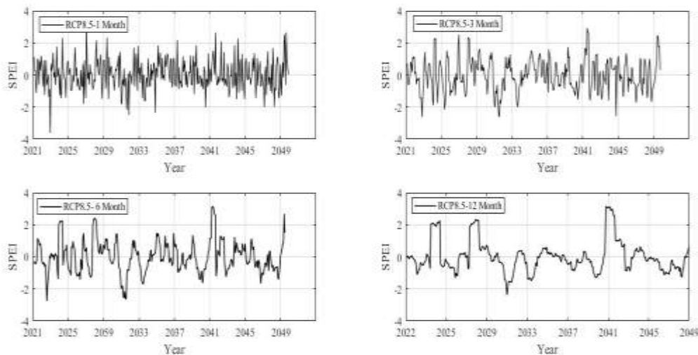
شکل (۷): تغییرات شاخص SPEI تحت سناریوی RCP8.5 در مقیاس های زمانی مختلف در دوره ۲۰۲۱-۲۰۵۰
