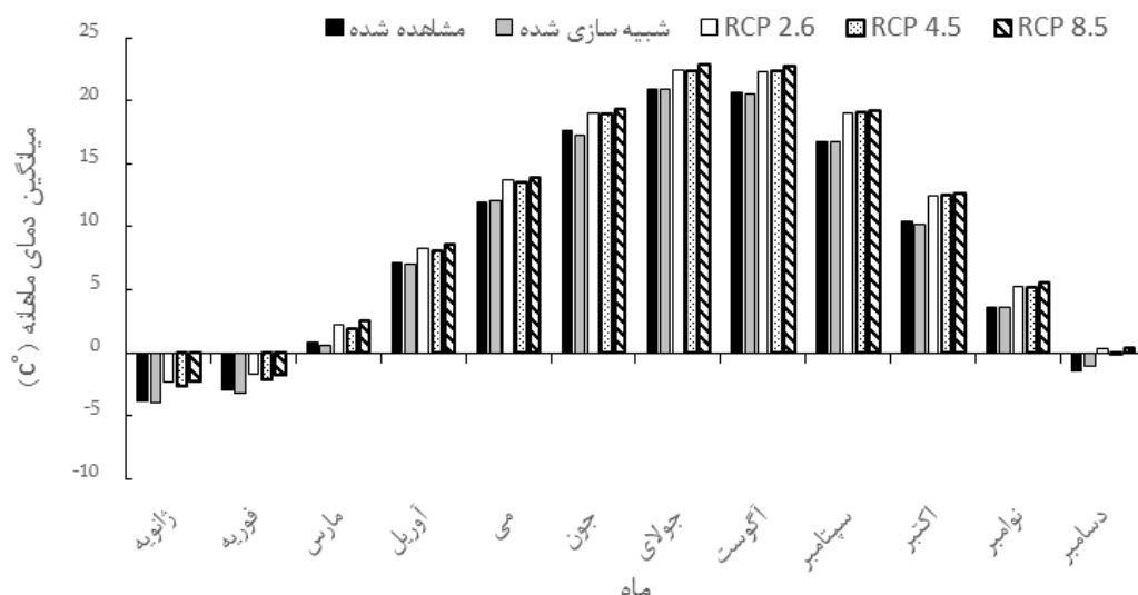
شکل (۳): میانگین دمای ماهانه ۱۹۹۲-۲۰۱۹ و ۲۰۲۱-۲۰۵۰ تحت سناریوهای RCP2.6، RCP4.5 و RCP8.5
