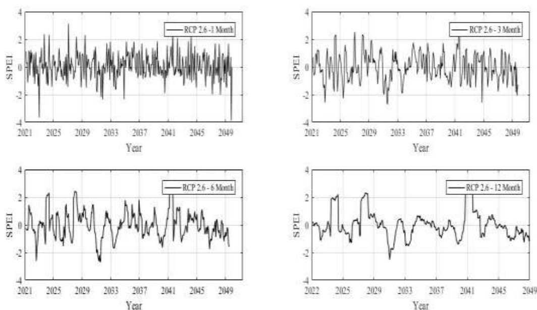
شکل (۵): تغییرات اساس شاخص SPEI تحت سناریوی RCP 2.6 در مقیاس‌های زمانی مختلف در دوره ۲۰۲۱-۲۰۵۰
