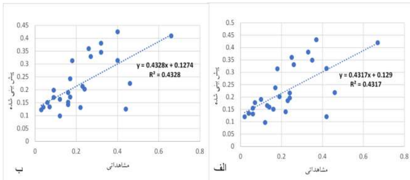
شکل (۳): الف: شاخص جریان کم (جریان کم / میانگین جریان در هر سال) و مشاهداتی و شبیه‌سازی شده براساس رگرسیون چندمتغیره ب: شاخص جریان کم (جریان کم / میانگین جریان در کل دوره) و مشاهداتی و شبیه‌سازی شده براساس رگرسیون چندمتغیره (تداوم ۶۰ روز)
