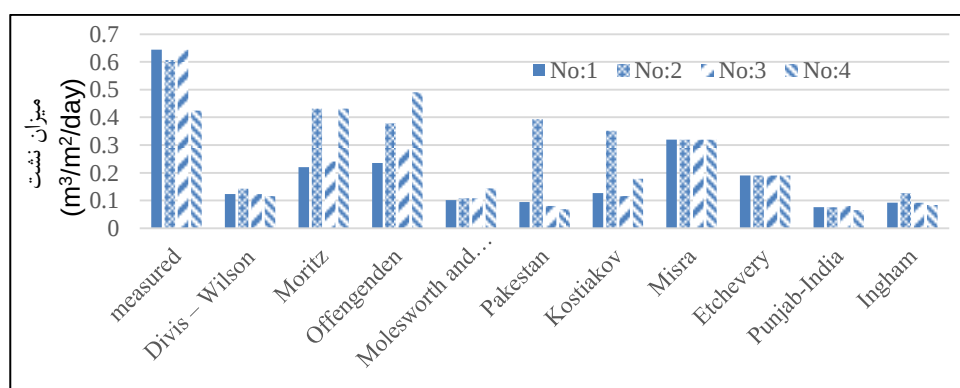
شکل (۷): مقایسه برآورد نشت آب از روش‌های تجربی با اندازه‌گیری انجام‌شده در کانال زرگران
