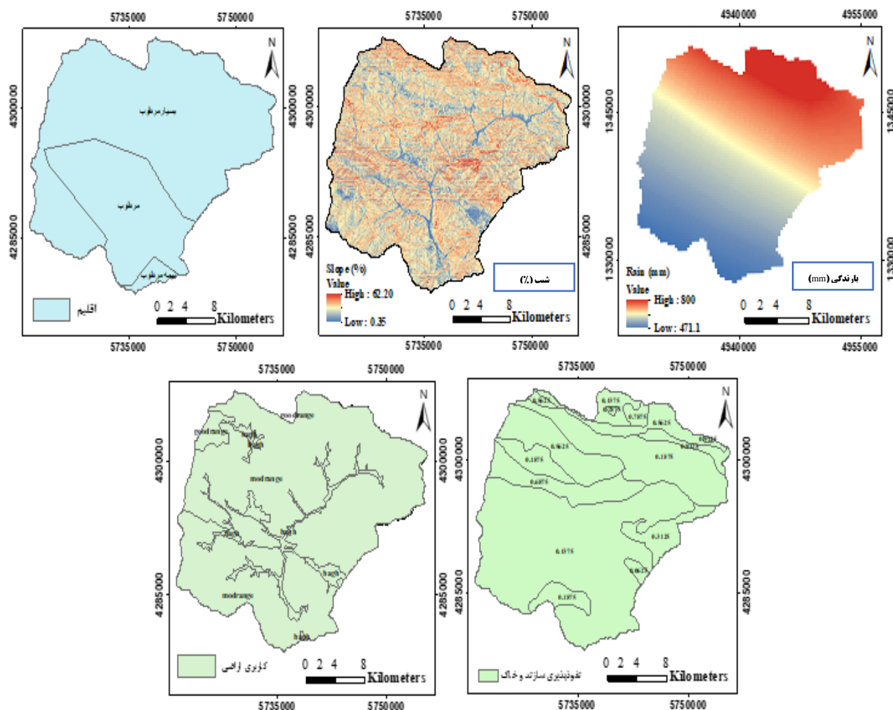
شکل (۲): نقشه‌ی شیب، اقلیم، بارندگی، کاربری اراضی و نفوذپذیری سازند و خاک در حوضه لتیان
