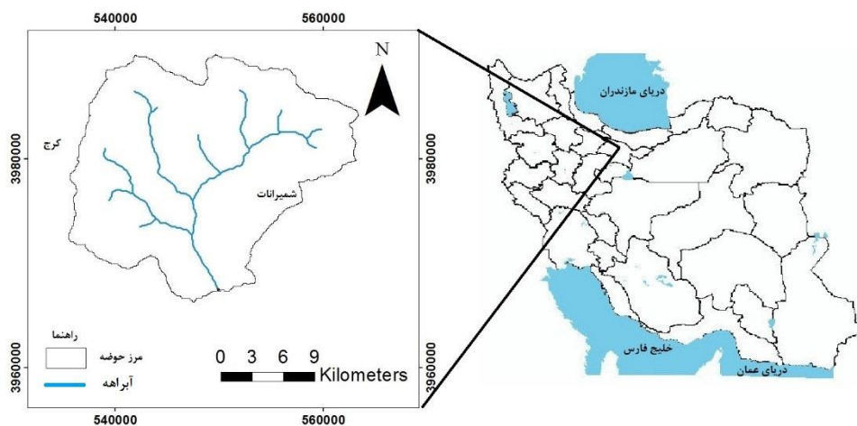
شکل (۱): موقعیت حوزه آبخیز لتیان
