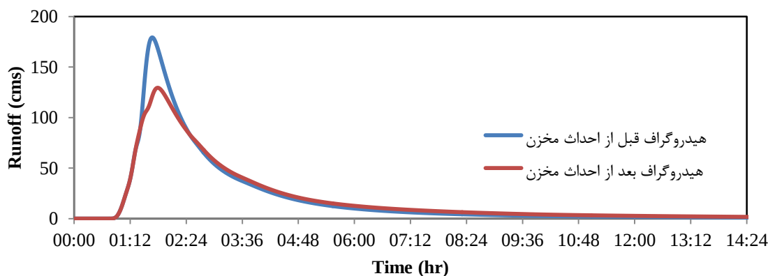
شکل ۶- هیدروگراف رواناب تولیدی در خروجی مسیل اقبال شرقی با سه مخزن (دوره بازگشت ۵۰ ساله)
