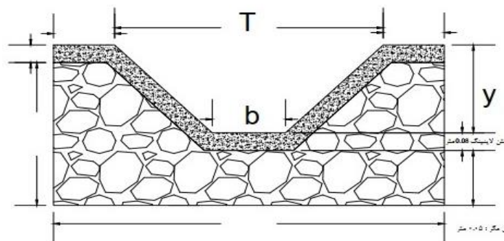
شکل ۲- مقطع کانال دوزنقه‌ای
