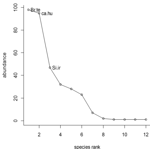
شکل (۳): منحنی رتبه-وفور گونه‌ای در مرتع چرا شده (سمت چپ) و قرق (سمت راست)
