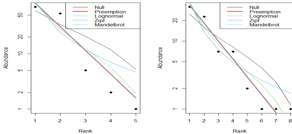
شکل (۷): پنج مدل برازش یافته با توزیع وفور گونه‌ای در سال خشک در مرتع تحت چرا (سمت چپ) و قرق (سمت راست)
