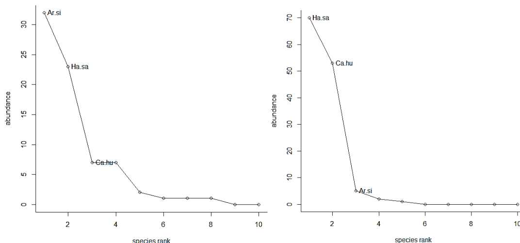
شکل (۶): منحنی رتبه-وفور گونه‌ای در مرتع چرا شده (سمت چپ) و قرق (سمت راست)
