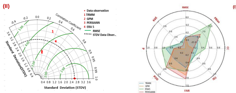
شکل ۵- تغییرات متوسط شاخص‌های آماری در سطح محدوده مورد مطالعه (I) و دیاگرام تیلور (II)
