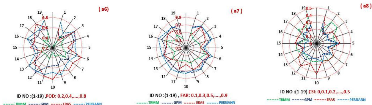
شکل ۳- تغییرات مقادیر شاخص‌های طبقه‌بندی بارندگی روزانه ایستگاه‌های باران سنج ثبات محدوده مورد مطالعه Figure 3- Changes in the values of daily rainfall classification indices of the stability rain gauge stations of the studied area
