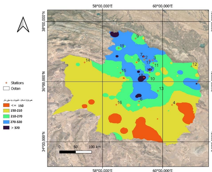
شکل ۱- نقشه متوسط بارش استان خراسان رضوی (۹۹-۱۳۶۹) و پراکندگی مکانی ایستگاه‌های باران سنج ثبات نیرو
