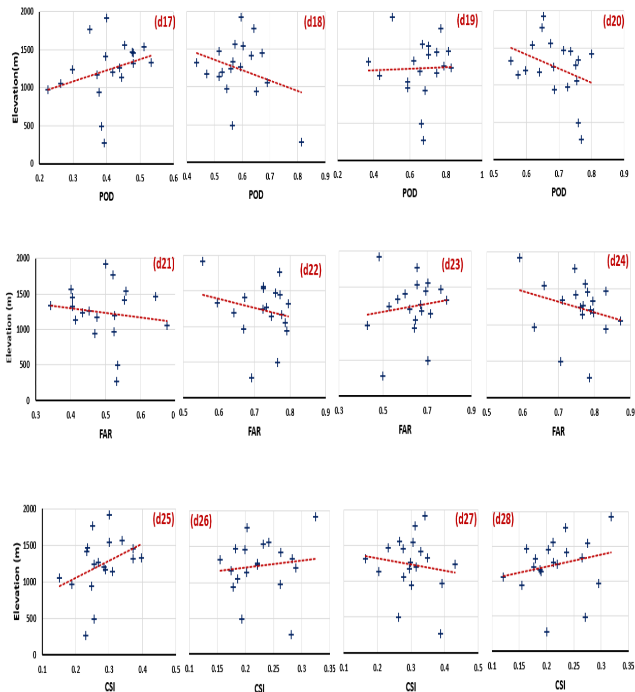
ادامه شکل ۶- تغییرات شاخص‌های آماری و عملکرد بارندگی روزانه محصولات ماهواره‌ها و سنجنده‌های با ارتفاع در محدوده مورد مطالعه Continued Figure 6- Changes in statistical indicators and daily rainfall performance of satellites and height gauges in the studied area
