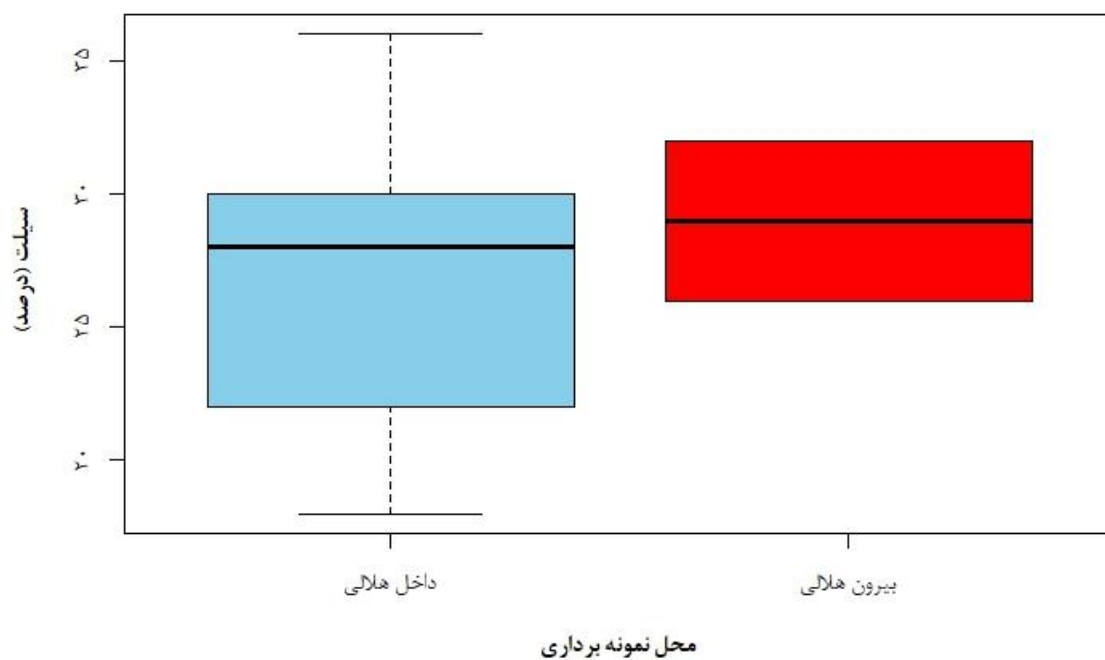
شکل ۱۵- مقایسه میزان سیلت خاک در داخل و بیرون هلالی
