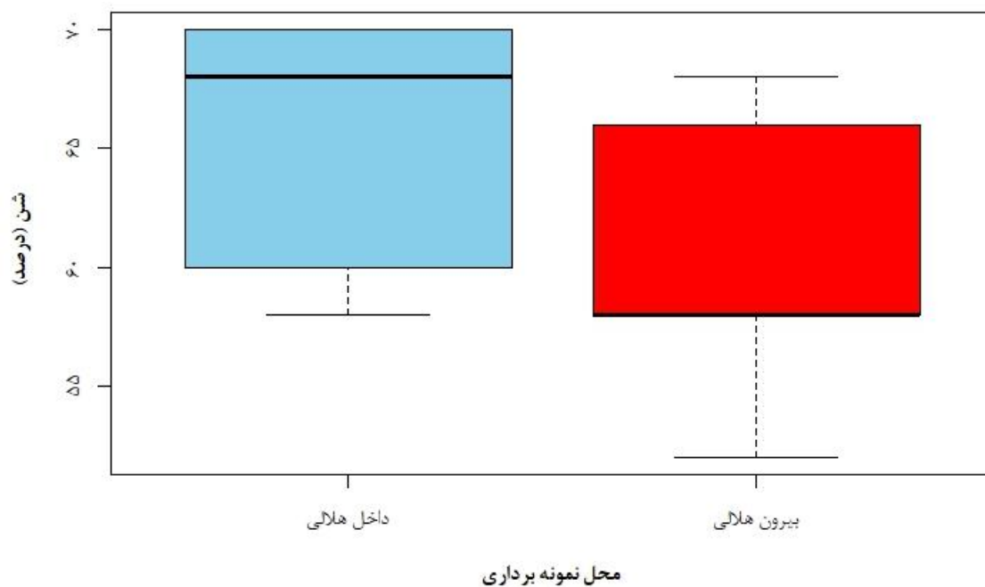
شکل ۱۴- مقایسه میزان شن خاک در داخل و بیرون هلالی
