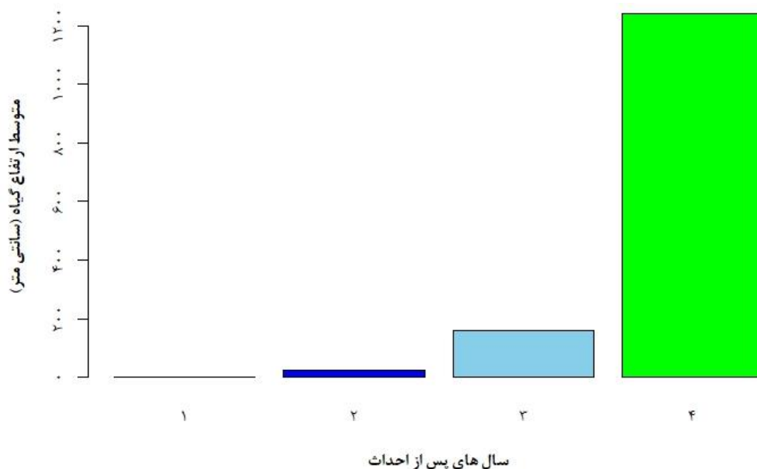
شکل ۴- تغییرات میانگین ارتفاع گیاه تاغ در سال‌های مورد مطالعه
