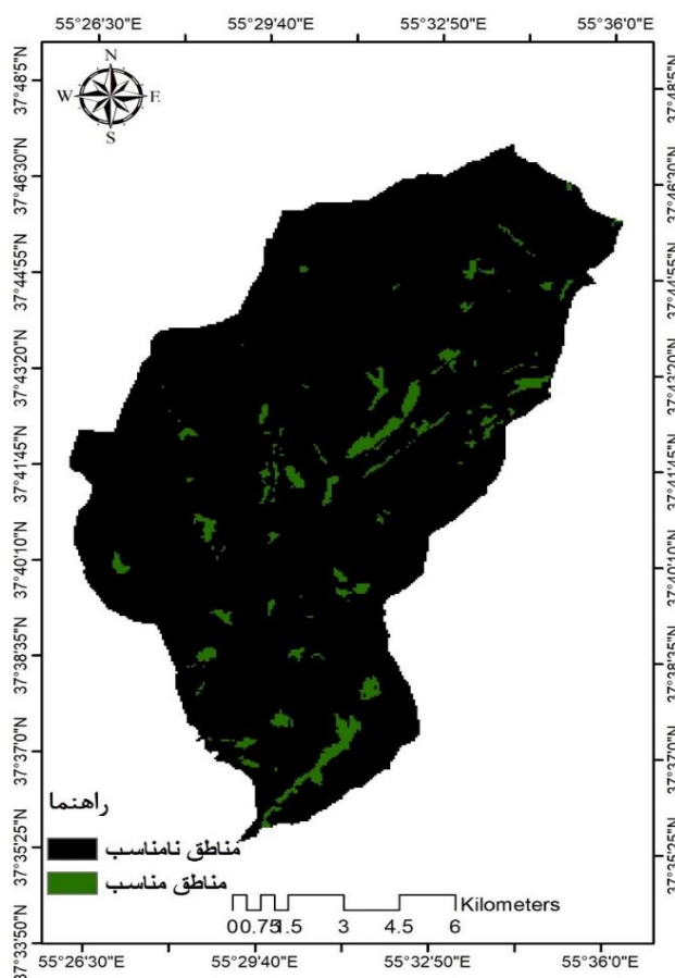
شکل ۹- محدوده‌های دارای توانایی بالقوه استحصال آب باران در حوزه آبریز قویجق
