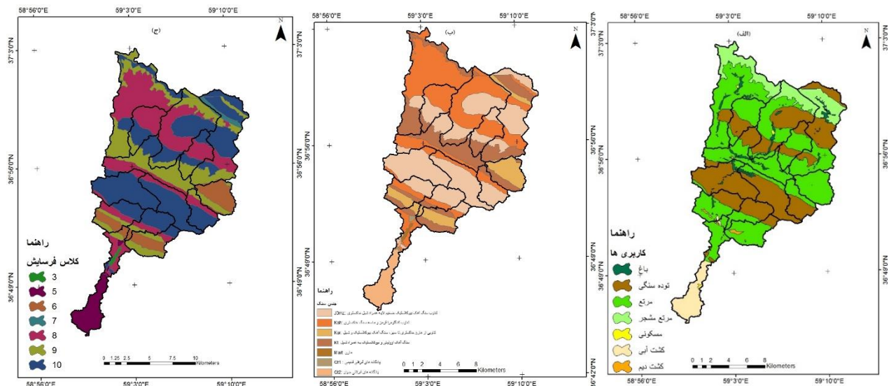
شکل ۳- نقشه کاربری اراضی (الف) سنگ‌شناسی (ب) و فرسایش (ج) حوزه آبخیز رادکان
