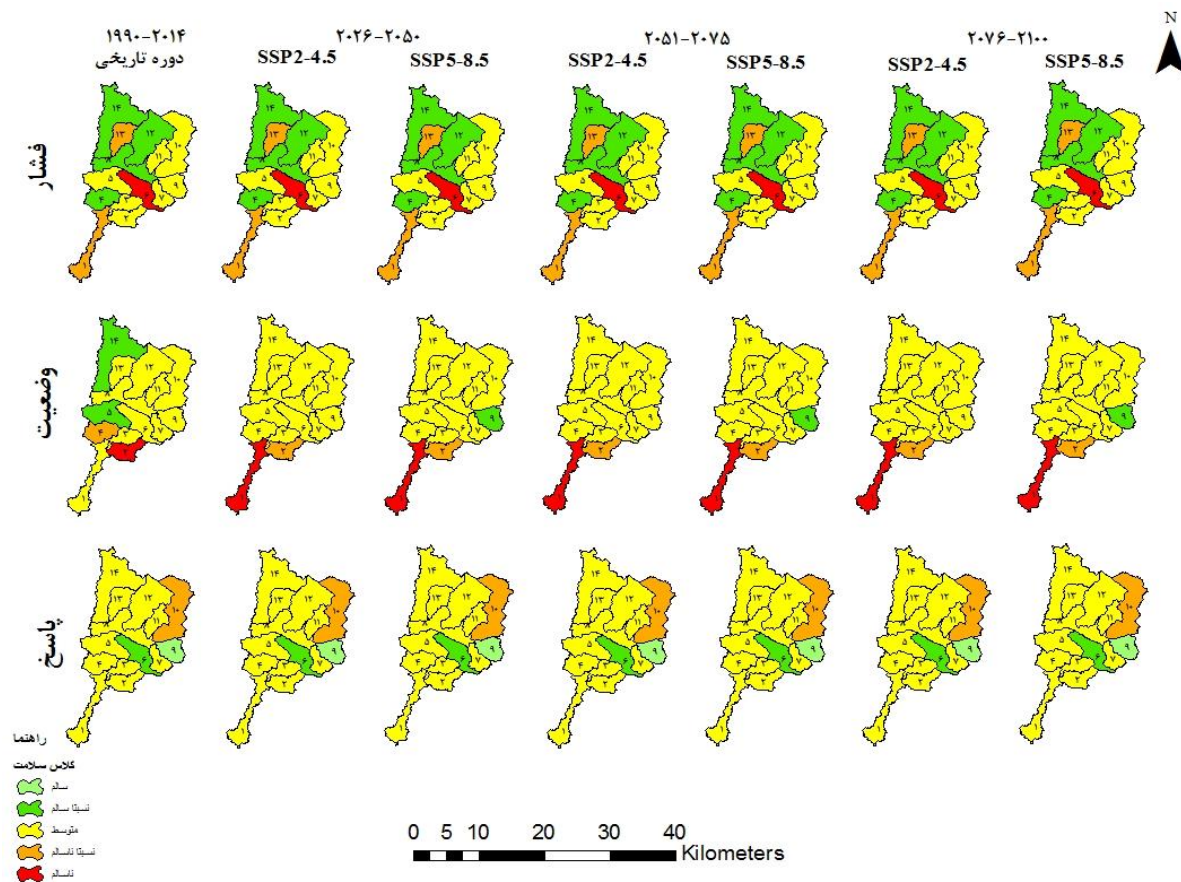
شکل ۵- تغییرات شاخص های فشار، وضعیت و پاسخ در دوره تاریخی و دوره های زمانی آینده تحت دو سناریو
