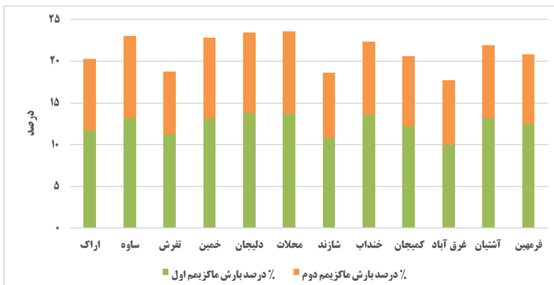
شکل ۴- درصد اولین و دومین حداکثر بارش ۲۴ ساعته نسبت به بارش سال زراعی در دوره آماری
