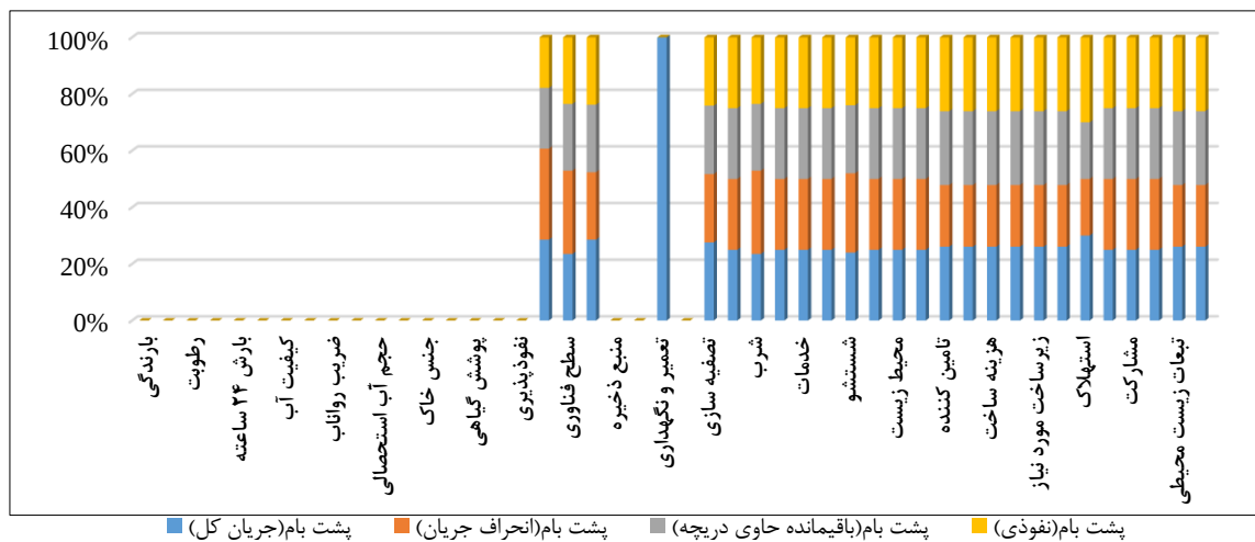
شکل ۵- نتیجه وزن دهی به معیارهای ارزیابی روش‌های پشت‌بام جهت جمع‌آوری آب باران
