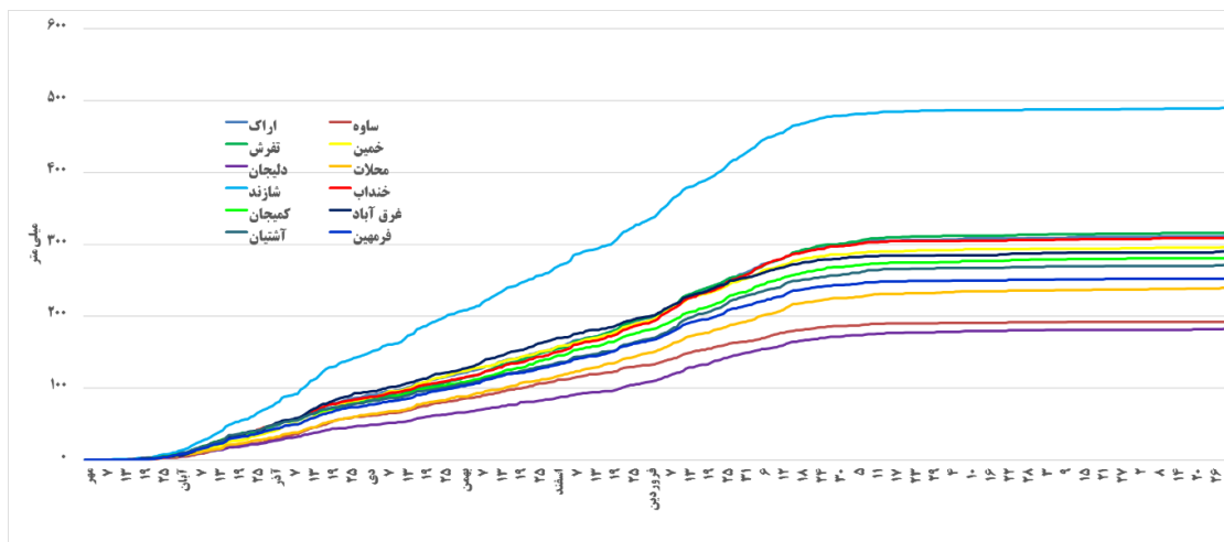
شکل ۳- نمودار تجمعی بارندگی ایستگاه‌های استان مرکزی
